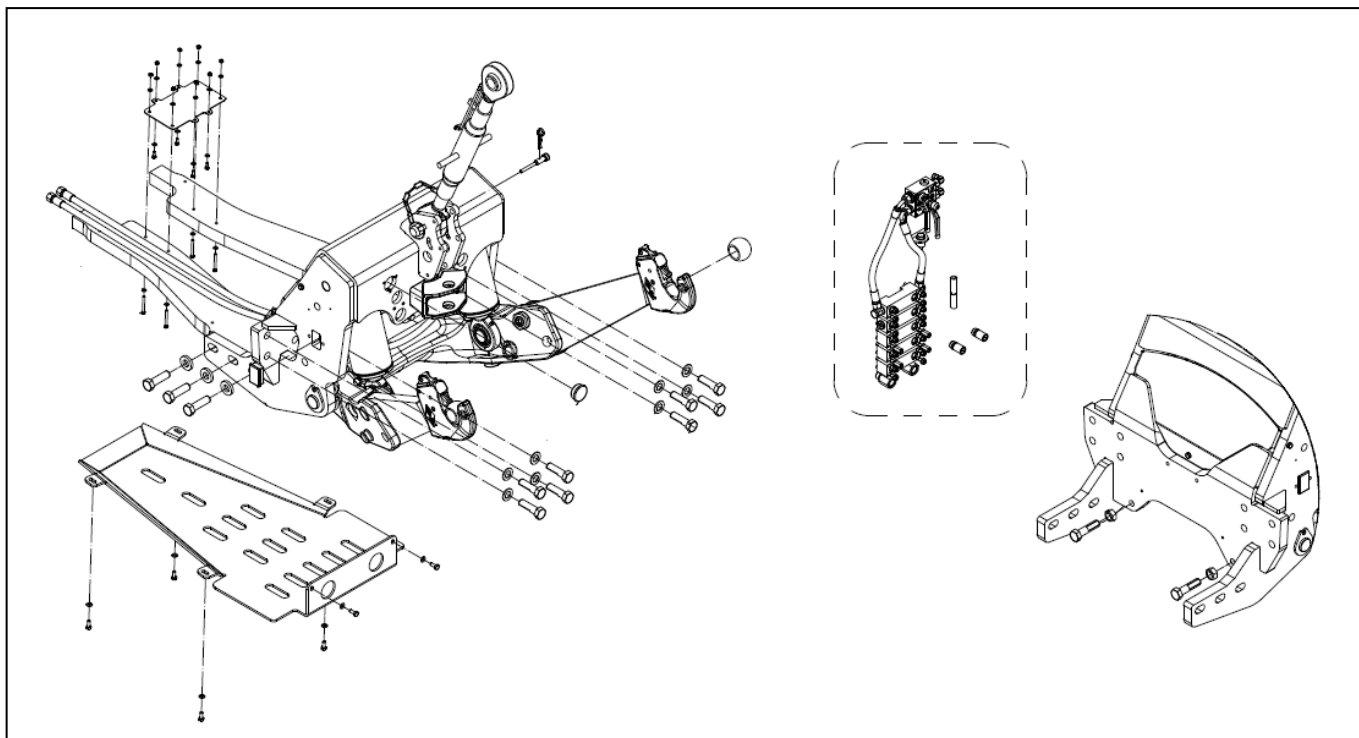
PZZ 50 kN (1410263)
