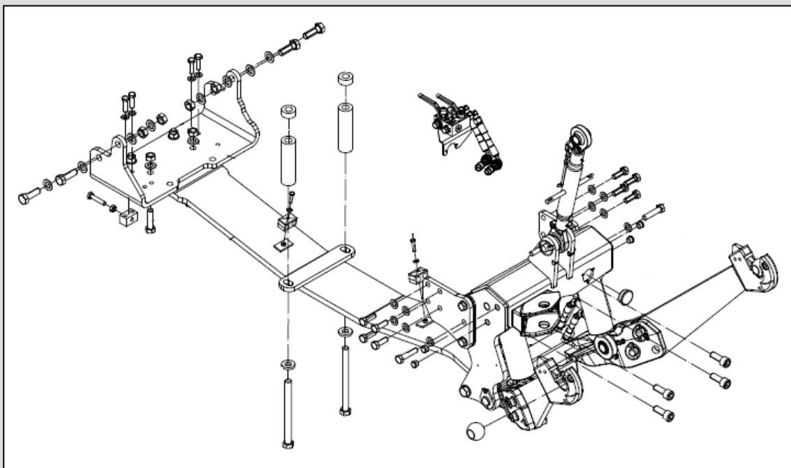
PZZ 18 kN (1410142)
