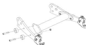
Výztuha spodních ram
