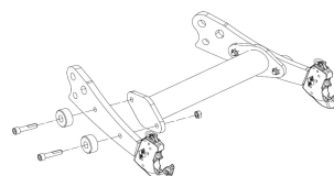
Výztuha spodních ramen
