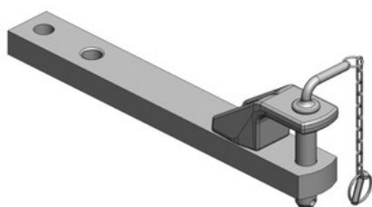
Tažná tyč, Cat. 3, kolík \varnothing 38mm
