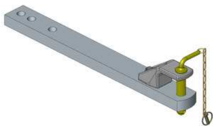
Tažná tyč, Cat. 2, kolík \varnothing 31 mm
