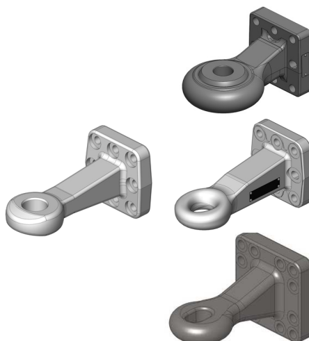
Tažná tyč, Cat. 3, kolík \varnothing 38mm
