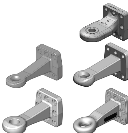
Tažná tyč, Cat. 2, kolík \varnothing 31 mm
