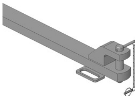
Tažná tyč, Cat. 4, kolík \varnothing 50 mm
