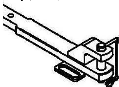
Tažná tyč, Cat. 5, kolík \varnothing 70 mm
